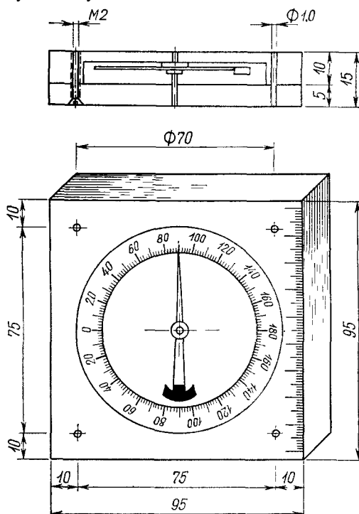
Рис. 53. Угломер Рихтера с утяжеленной стрелкой
