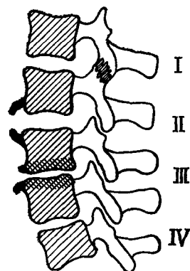
Рис. 173. Дегенеративные изменения в позвоночнике: I — спондилартроз, II — деформирующий спондилоз, III — остеохондроз, IV — межпозвонковый хондроз (сужение диска)
